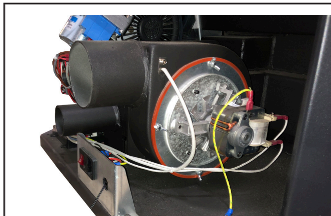
Figure 26 Ventilateur d'échappement du modèle PSBF66W
